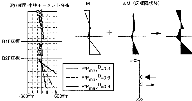
図-5 B2F中柱・逆せん断力の作用メカニズム
