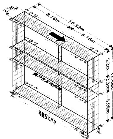
図-1 3次元静的非線形解析モデル
