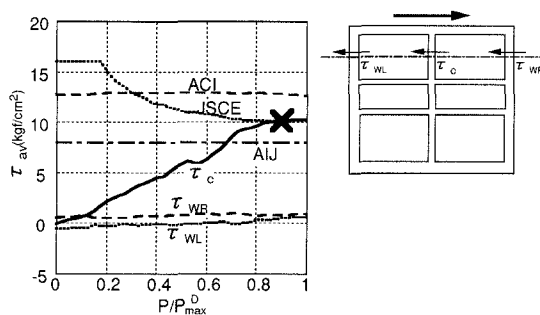
図-3 せん断応力度-荷重関係 (B1F中腹)
