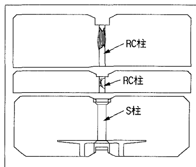
図-2 中柱の被害状況
