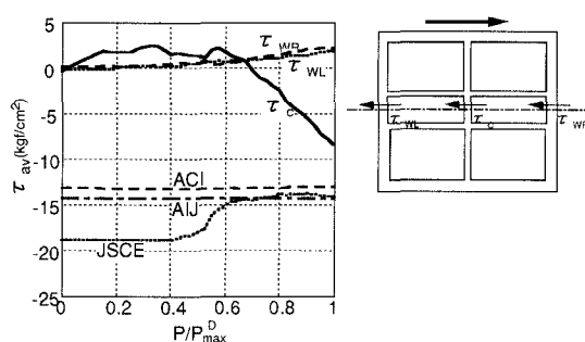
図-4 せん断応力度-荷重関係 (B2F中腹)
