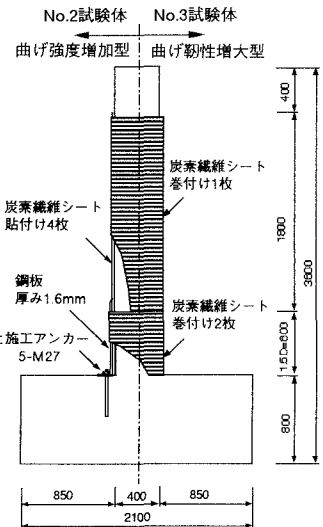
図-2 補強概要
