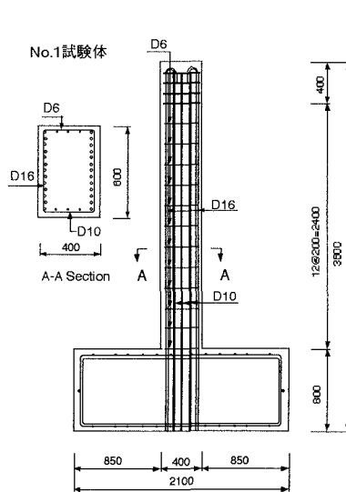
図-1 試験体の形状・寸法および配筋
