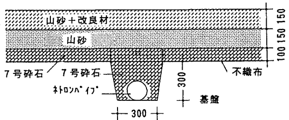
図4 ラグビーグラウンド断面図 ～植生基盤構造～
