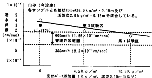
図2 完全バークと透水係数との関係
