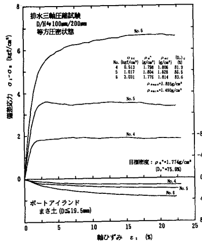
図-3 (a) まさ土 ( D_r^* \approx 45\% )
