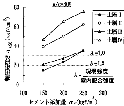
図-3 配合試験結果(高炉セメントB種)。
