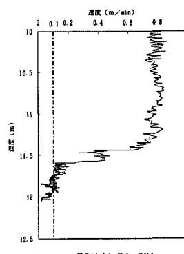
図-5 貫入速度と深さの関係
