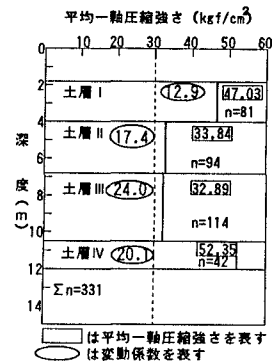
図-6 一軸圧縮試験結果
