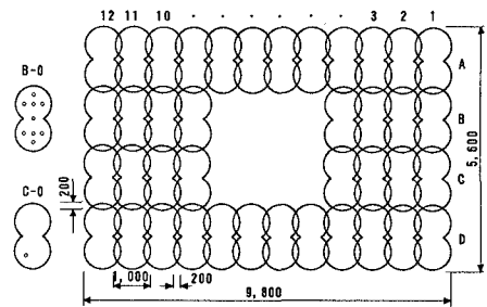
図-4 改良柱の配置
