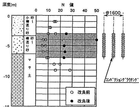
図-1 土質柱状図
