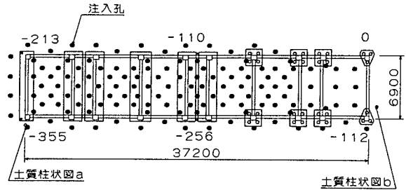
図－3 基礎平面図
