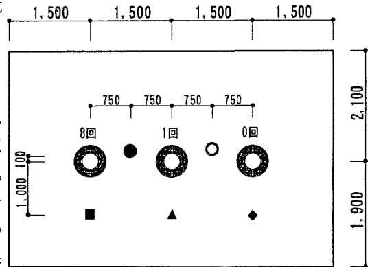
図-3 試験杭打設位置および地盤調査位置
