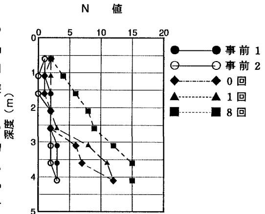
図-4 事前事後のN値の比較
