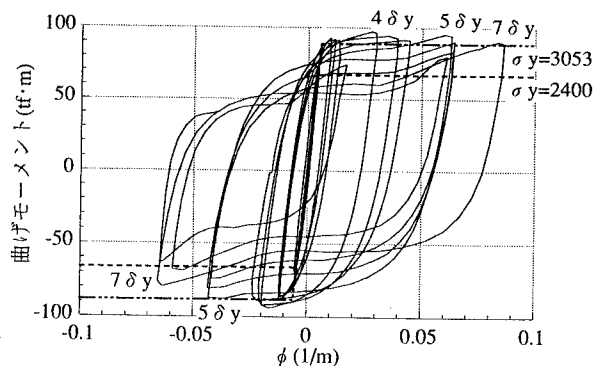
図7 曲げモーメントと曲率の関係(CASE2)
