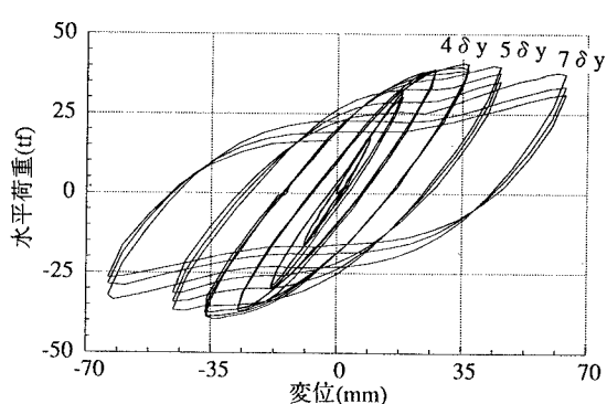
図5 水平変位-水平荷重関係(CASE2)
