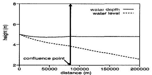
図 5: 40200 sec での水位の変化
