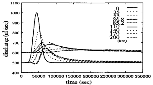
図 4: Case 2 における流量の時間的変化
