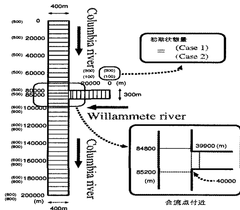
図 2: Columbia-willamette 川の形状
