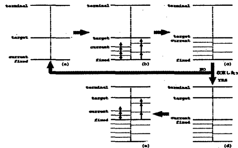
図1: 反復計算の進め方
