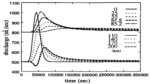
図 3: Case 1 における流量の時間的変化
