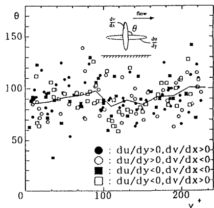
図-7 高せん断領域の交差角
