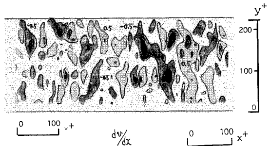
図-6 鉛直方向変動速度勾配分布
