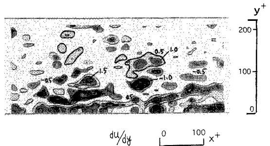
図-5 流れ方向変動速度勾配分布
