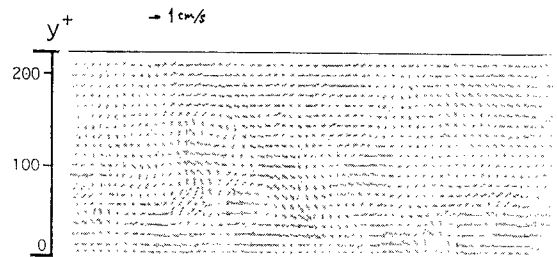
図-2 変動速度ベクトル
