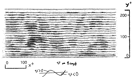
図-4 鉛直方向変動速度分布
