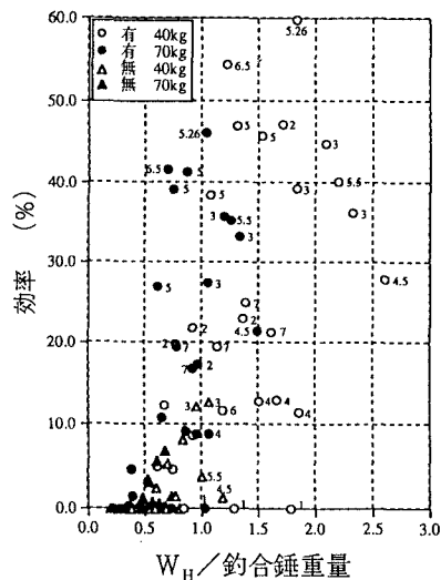
図-3 効率と W_H /釣合錘重量の關係
