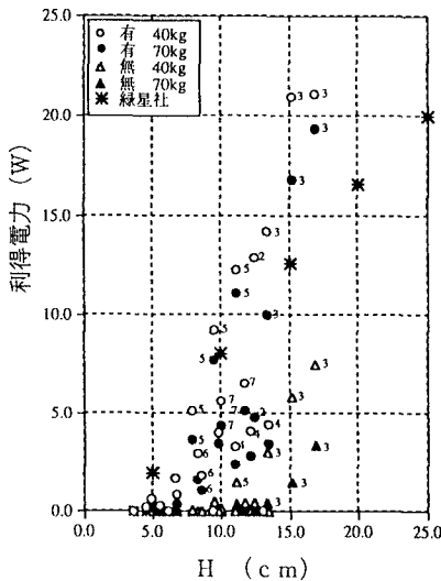
図-2 利得電力と波高の關係
