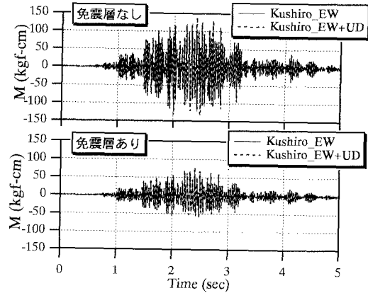
図4 曲げモーメントの応答波形 (釧路波、底版外側コーナー)
