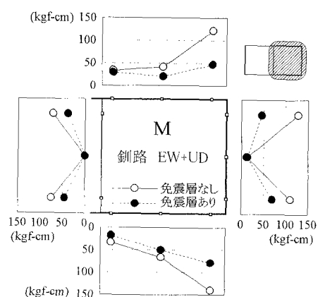
図6 曲げモーメントの最大値分布 (水平・上下方向加振)
