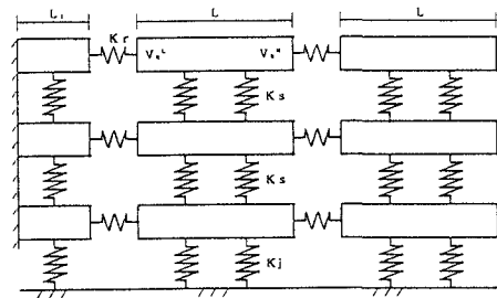
図1 解析モデル
