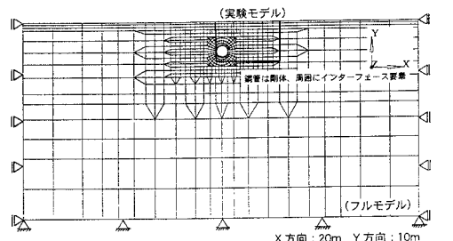
図3 解析用2次元FEMモデル
