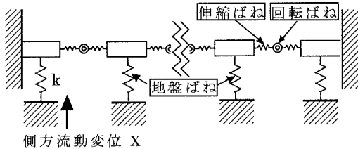
図5 パイプラインモデル
