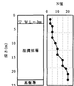
図1 地盤モデルの地層構成
