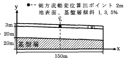
(a) 無対策モデル
