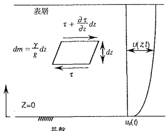
図-1 地盤震動の概念図
