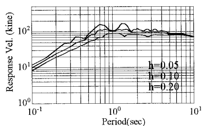
(b) 速度応答スペクトル
