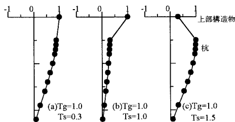
図5 振動モード
