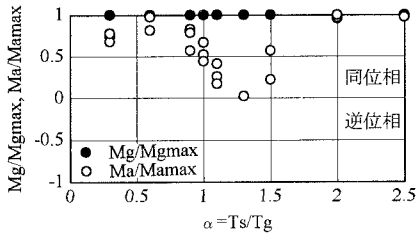
図3 地盤変位最大時刻での応答値
