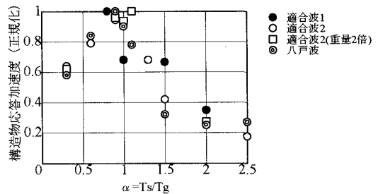
図6 T_s/T_g と応答加速度との関係
