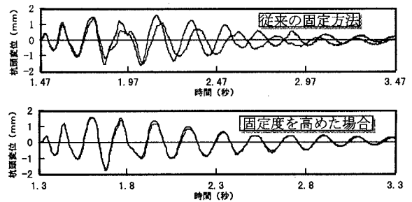
普通杭 2本 気中加振、杭頭重量 2.17kg 図-5 2本の普通杭の杭頭変位に現れた固定度の影響 （加振波は1995年兵庫県南部地震JMA神戸NS）
