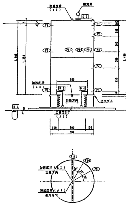
図-1 動揺振動モデル概要図 (モデル4)
