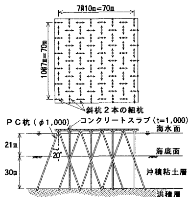
図1 斜杭式人工島
