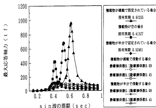
図3 sin波入力による共振曲線（周期－応答）
