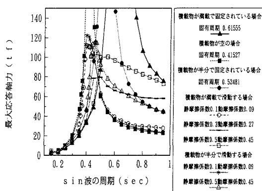
図4 sin波入力による共振曲線（周期－応答）
