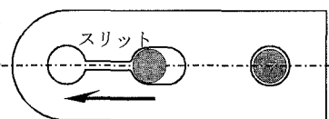
図2 スリットを持つ連結板
