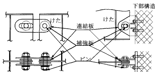
図1 連結板を用いる落橋防止装置
