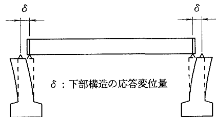
図-4 下部構造頂部の変位量
