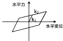
図-4 免震支承モデル
