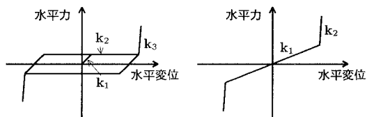
図-2 鋼製可動支承モデル 図-3 ゴム可動、水平反力分散支承モデル
