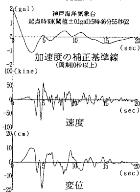
図-2 加速度の補正基準線と速度および変位波形 (EW成分)
