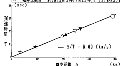
図-5 地震動の到達時間と震央距離
