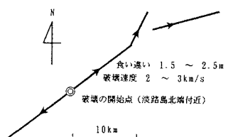
図-1 兵庫県南部地震の発生メカニズム 1)
