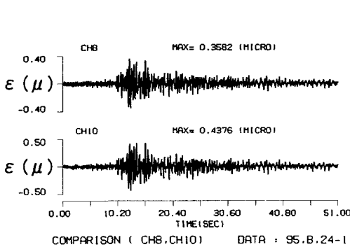
図-3 時刻歴波形
