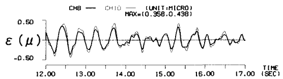
図-5 2波形の重ね書き（主要動部）
