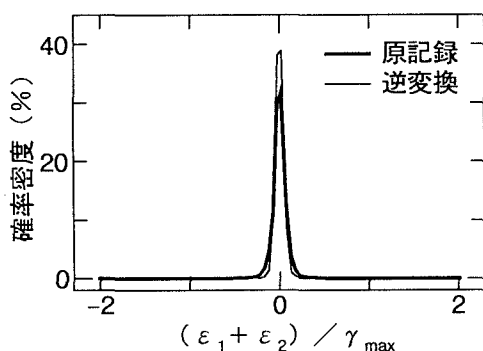
図－3 (\varepsilon_1 + \varepsilon_2) / \gamma_{max} の確率密度分布
