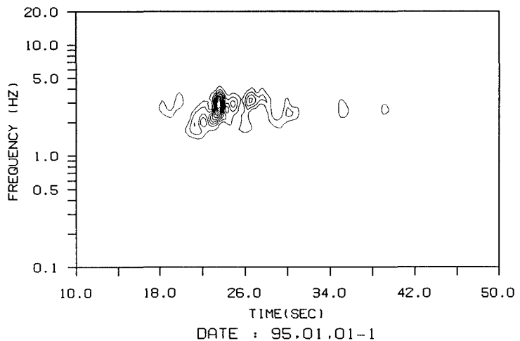
図－2 時間－振動数スペクトル
