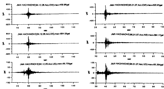
図3. 八戸測候所で加速度記録と加速度応答スペクトルの例（三陸はるか沖地震の本震と最大余震）
