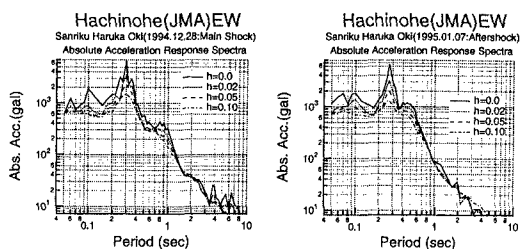
図3. 八戸測候所で加速度記録と加速度応答スペクトルの例（三陸はるか沖地震の本震と最大余震）
