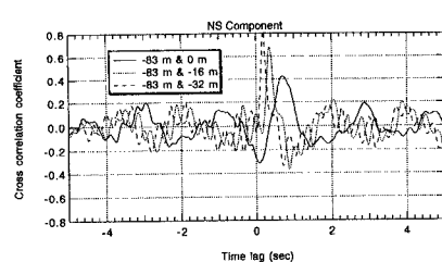
図3 相互相関係数（NS成分）
