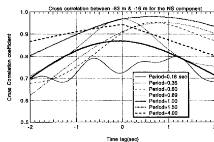
図5 非定常スペクトル振幅の相互相関係数
