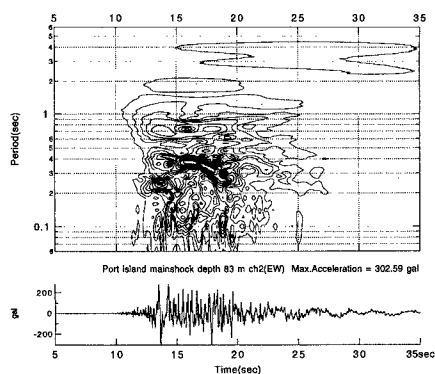
図4 非定常スペクトル（深さ83m、EW成分）
