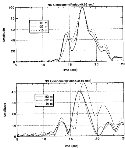
図6 各深さの非定常スペクトル振幅の同時時間軸プロット
