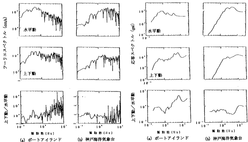
図2. 実地震波のフーリエスペクトル ならびに上下動と水平動の比
