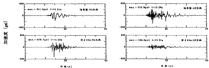
図1. ポートアイランドにおける地震動の加速度時刻歴
