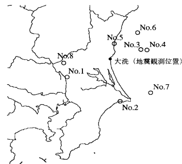
図-1 震源位置分布
