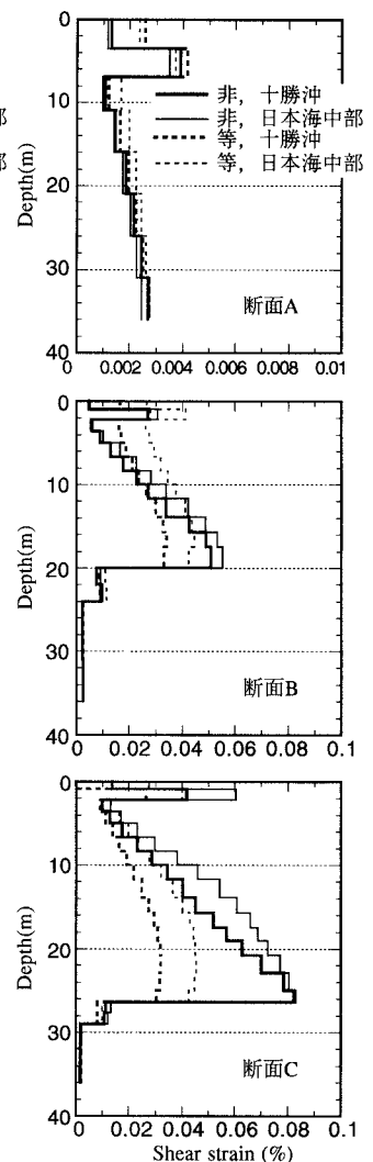
図4 最大せん断ひずみ分布
