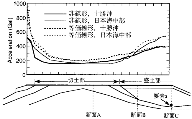
図2 地表面の最大加速度分布
