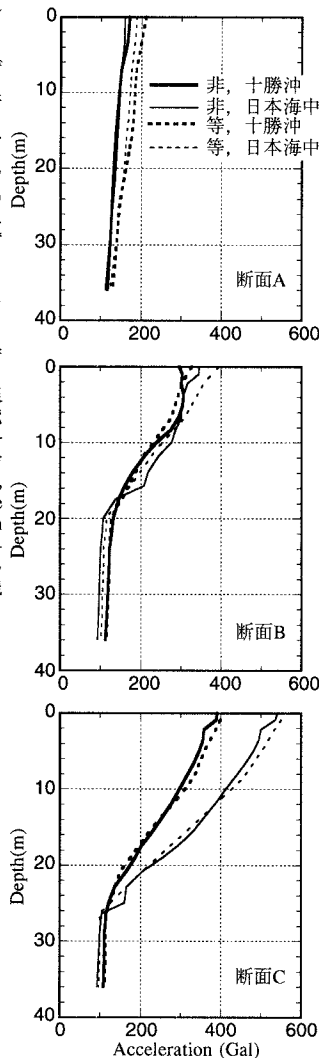
図3 最大加速度分布
