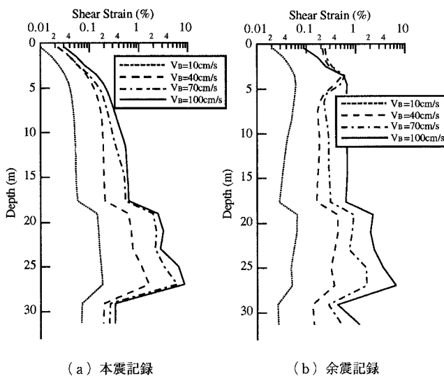
図－3 入力最大速度と最大せん断ひずみの鉛直分布の関係
