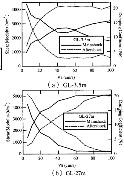
図－4 入力最大速度とG、hの関係
