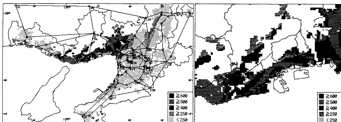
図-4 推定した広域加速度分布
