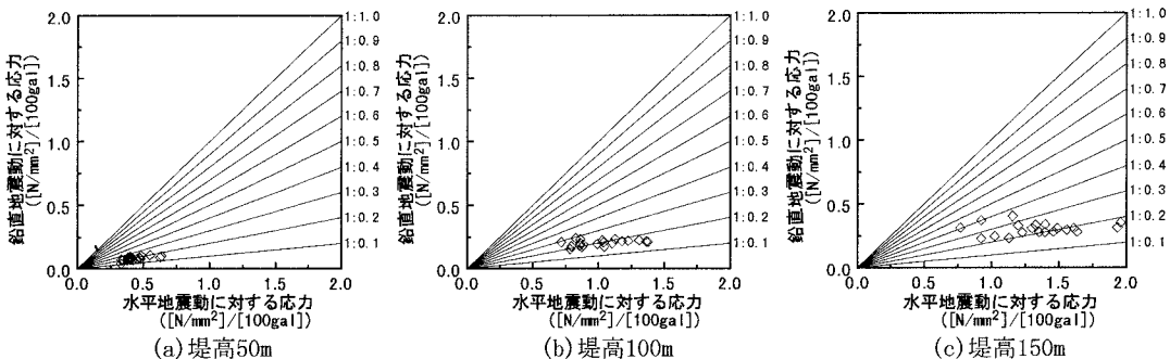
図-4 水平および鉛直地震動による応力の比較（鉛直地震動：実測水平加速度波形）
