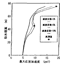
図-6 最大応答加速度分布
