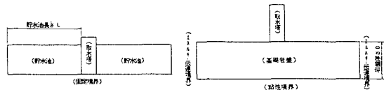
図-1 解析モデルの概略図
