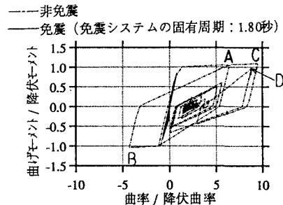
図-4 橋脚基部の載荷履歴（神戸波入力時）
