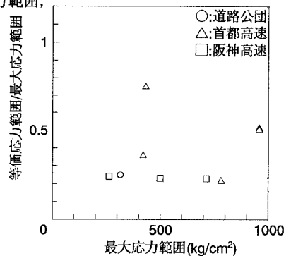
図3 \sigma_{r, max} と \sigma_{eq} / \sigma_{r, max} の関係
