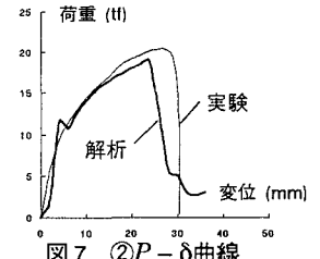
図7 ②P-δ曲線
