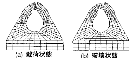
図8 ③耐震連結板B (高速載荷) の解析結果
