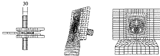
図5 ②③耐震連結板Bの解析モデル
