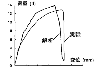
図4 ①耐震連結板AのP-δ曲線
