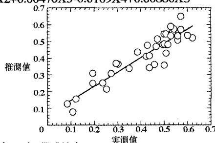
図-4 回帰式の内容及び回帰式精度
