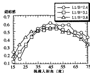
図-5 L1/Bの変化による錯綜感の特性変化
