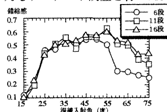
図-3 ケーブル段数の変化による錯綜感の特性変化
