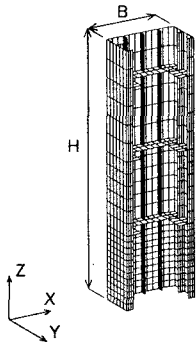
図-1 立体モデル
