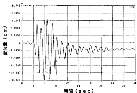
図-6 脚上部地震応答変位
