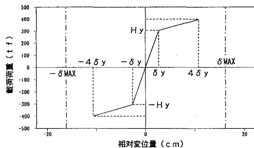
図-5 復元力モデル
