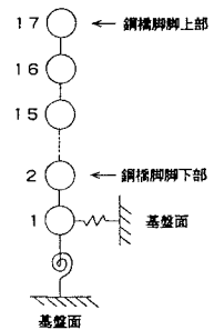
図-4 地震解析モデル
