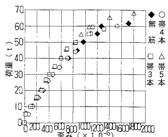
図3 帯鉄筋の形状別 最大荷重-歪み グラフ
