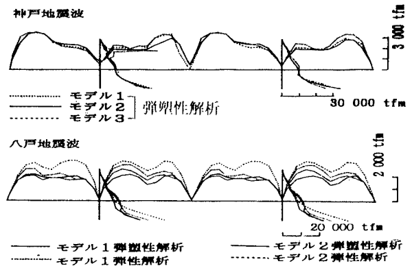
図-5 応答最大曲げモーメント
