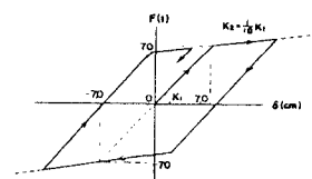
支持ばね-2
