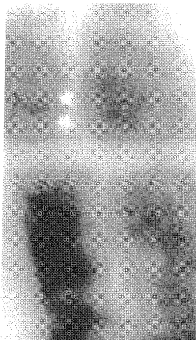
写真-2 ひび割れ (X線フィルム)
