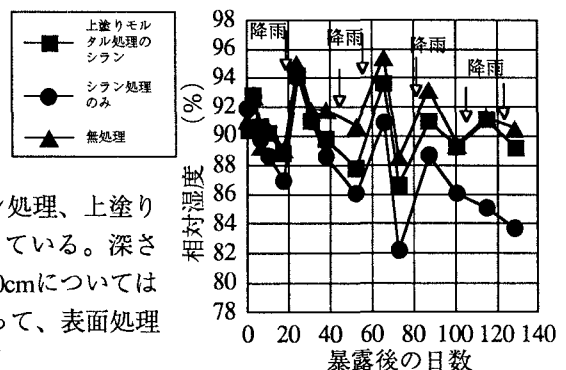
図6 深さ5cmでの相対湿度の経時変化
