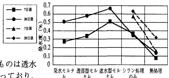
図4 上塗りモルタルの影響
