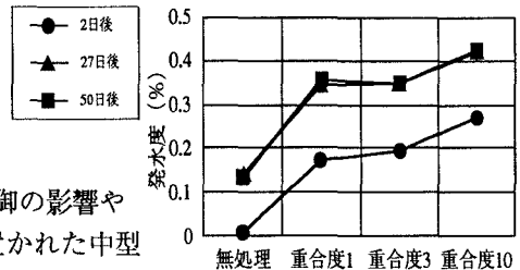
図1 重合度の影響
