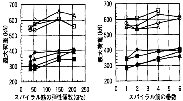
図3 最大荷重
