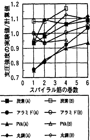
図4 支圧強度の実験値/計算値
