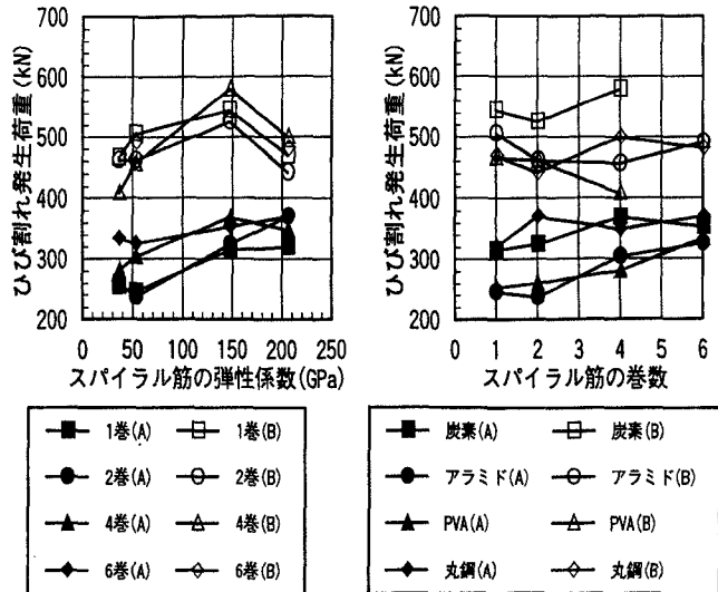
図2 ひび割れ発生荷重
