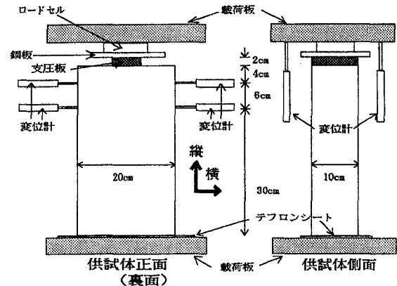
図 1 載荷状況
