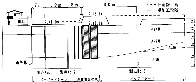
图-1 施工概要
