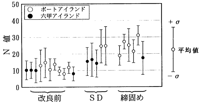
図-3 各工法のN値の分布
