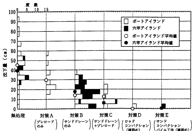
図-4 対策工法と沈下量の関係
