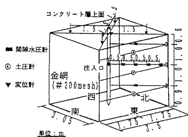
図-2 実験土槽
