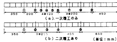
図2. ひずみ計測断面
