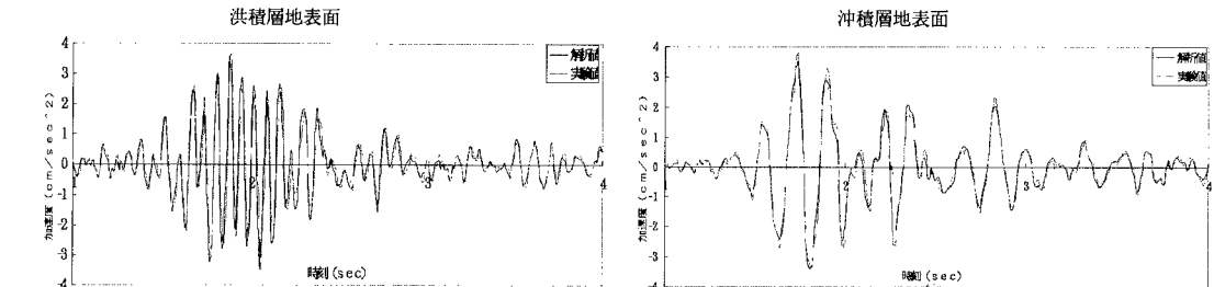
図6. 加速度の時刻歴
